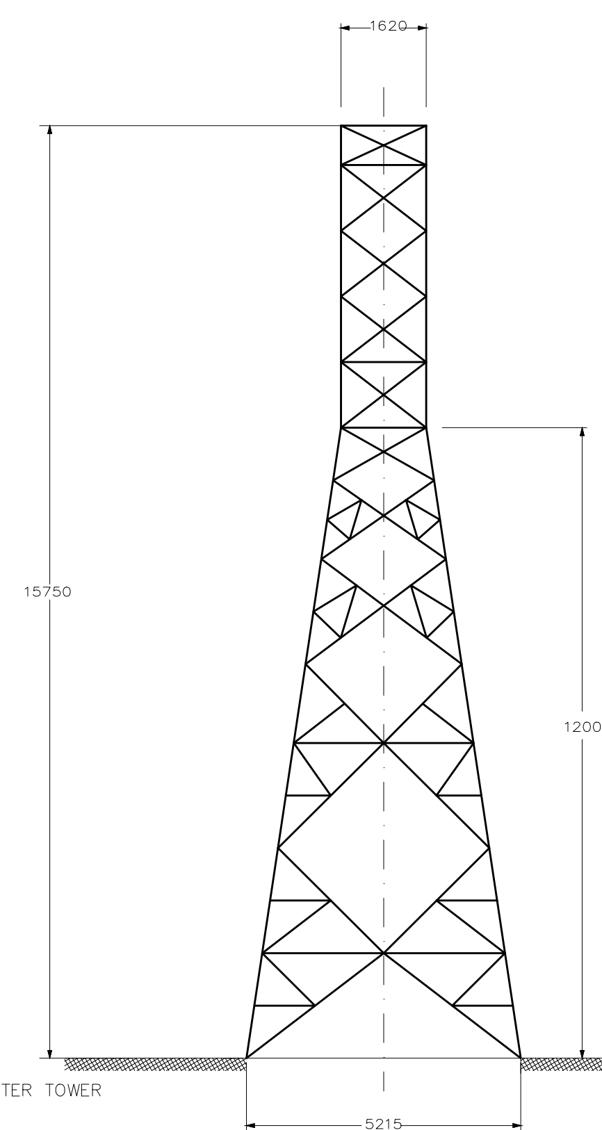
TYPICAL LONGITUDINALFACE
